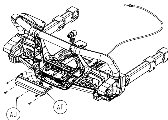
Figure 90 – Retirer l'ensemble de câble du module d'éclairage
