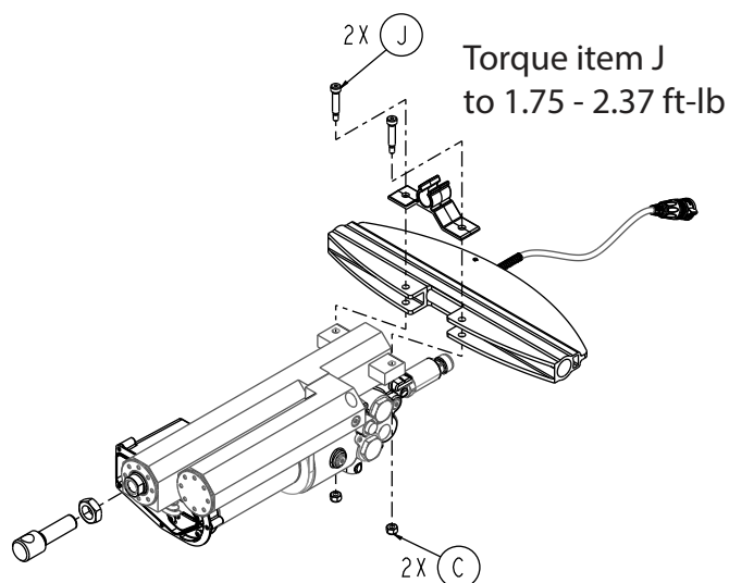
Figure 44 – Retirer les boulons et les écrous de l'ensemble actionneur
