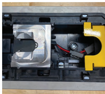
Ábra 15 – Csatlakozók helyei
