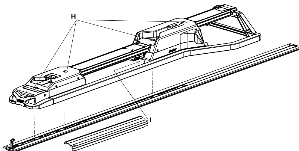
Figur 17 – Anslut fästeanordningen
