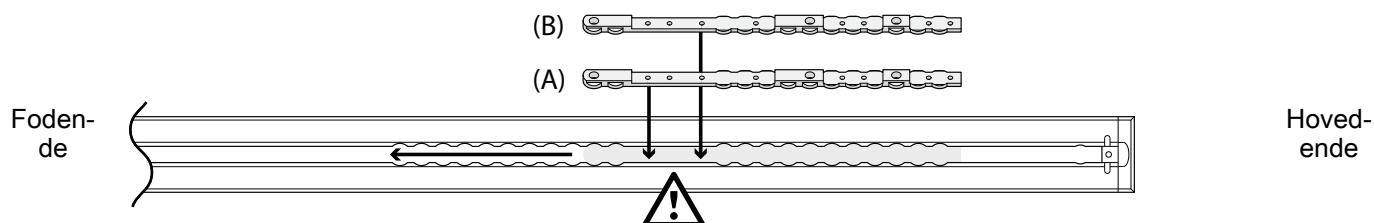
Figur 5 – Klampens installationssted
