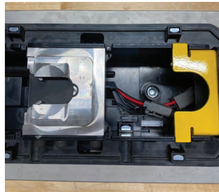
Kuva 15 – Liittimien sijainti
