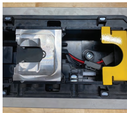
Afbeelding 15 – Connectorlocaties
