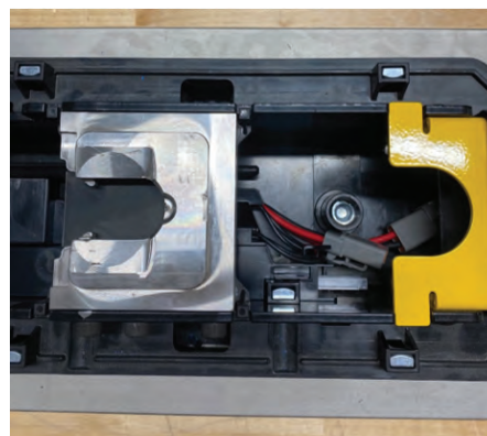
Figur 15 – Konnektorplaceringer
