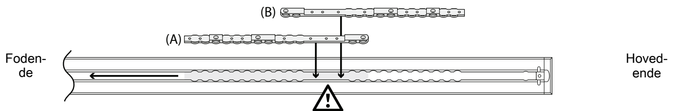
Figur 7 – Klampens installationssted
