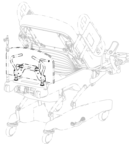
Figura 53 – Cambio de la cabecera
