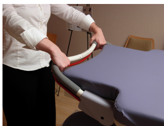
Figure 40 – Serrage de la poignée de déverrouillage de la section pieds et de la barre de verrouillage
