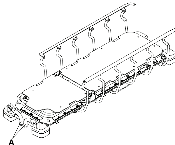
Rysunek 8 – Składanie uchwytów po stronie wezglowia
