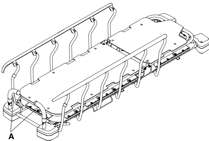
Figur 9 – Posisjonere skyvehåndtakene i fotenden
