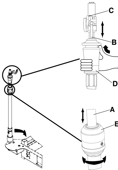
Afbeelding 13 – De permanent bevestigde drietrapsinzuigspaal positioneren
