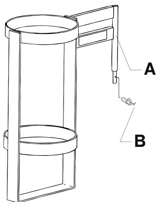
Figure 17 – Fixation du support pour bouteille d'oxygène
